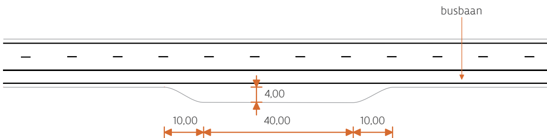
figuur 52: Pechhaven langs busbaan op Vlaamse hoofdwegen
