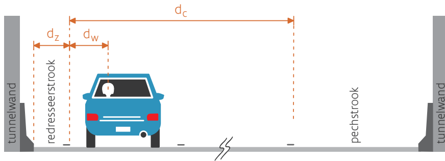
figuur 84: Schematiseringen voor bepaling wegverloopzicht
