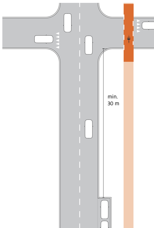
fig. 7: Onderbreking parkeerstrook
