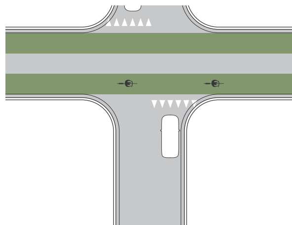
Fig. 2: Fietssuggestiestrook op een voorrangsweg
