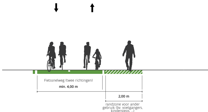
Fig. 2: Fietssnelweg met randzone voor ander gebruik
