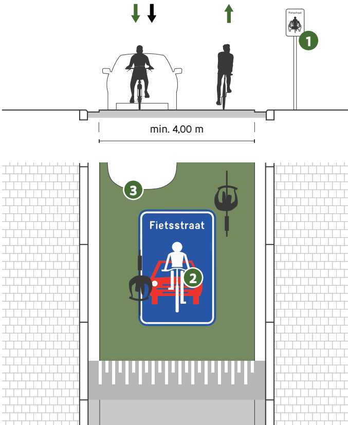
Fig. 2: Toegang tot een fietsstraat met BEV
