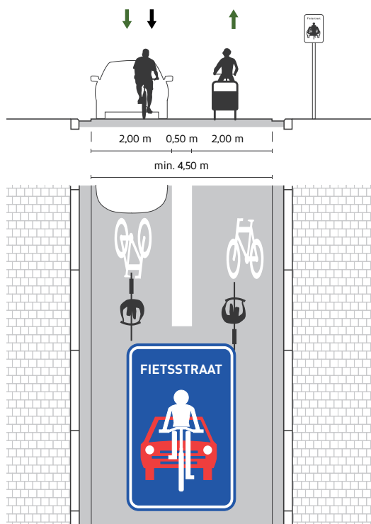
Fig. 5: Fietsstraat waarbij de fietsrijloper wordt aangeduid met markeringen.
