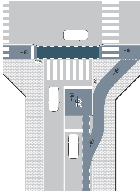
Fig. 1: Detailvoorbeeld bypass
