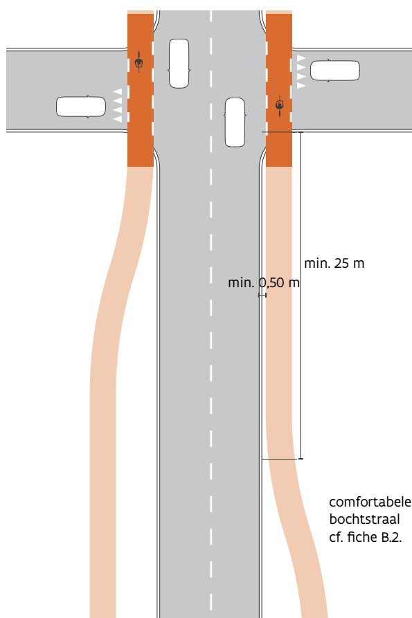
Fig. 3: Inbuigend eenrichtingsfietspad
