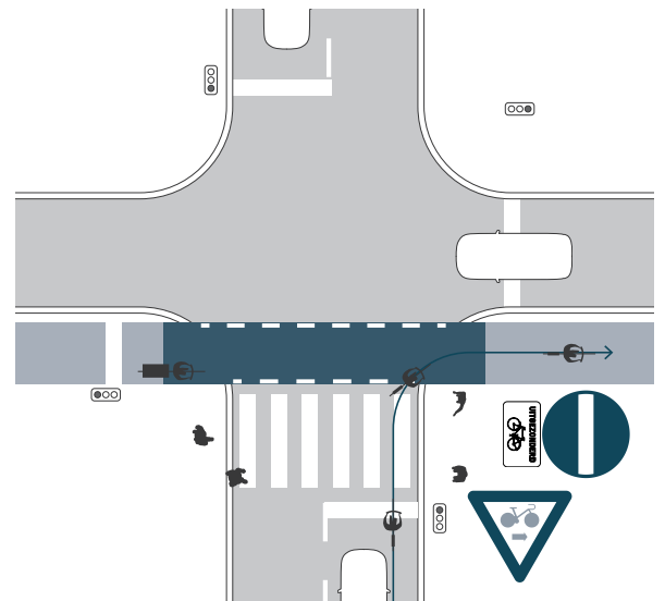
Fig. 4: BEV met fietspad in de rijrichting van de fietser
