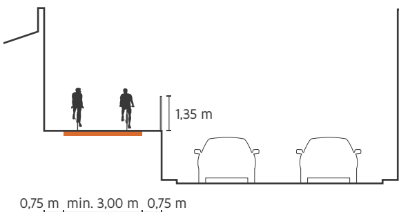
Fig. 1: Onderdoorgang op verschillende niveaus
