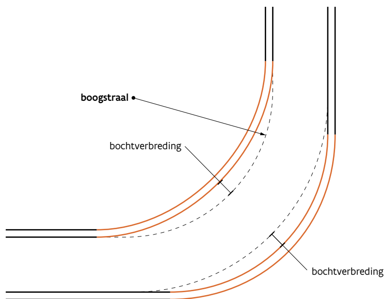
Fig. 1: Boogstraal en bochtverbreding ter hoogte van kruispunten en oversteekplaatsen (90°)
