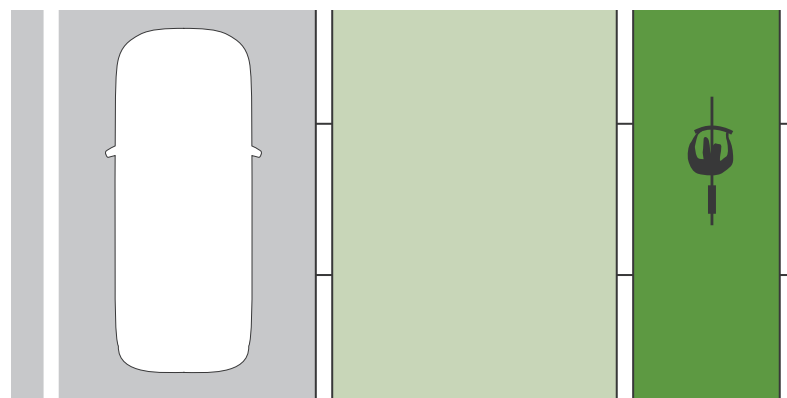
Fig. 2: Profiel vrijliggend eenrichtingsfietspad met een tussenstrook van 4,00 m bij een snelheidsregime van 90 km/u
