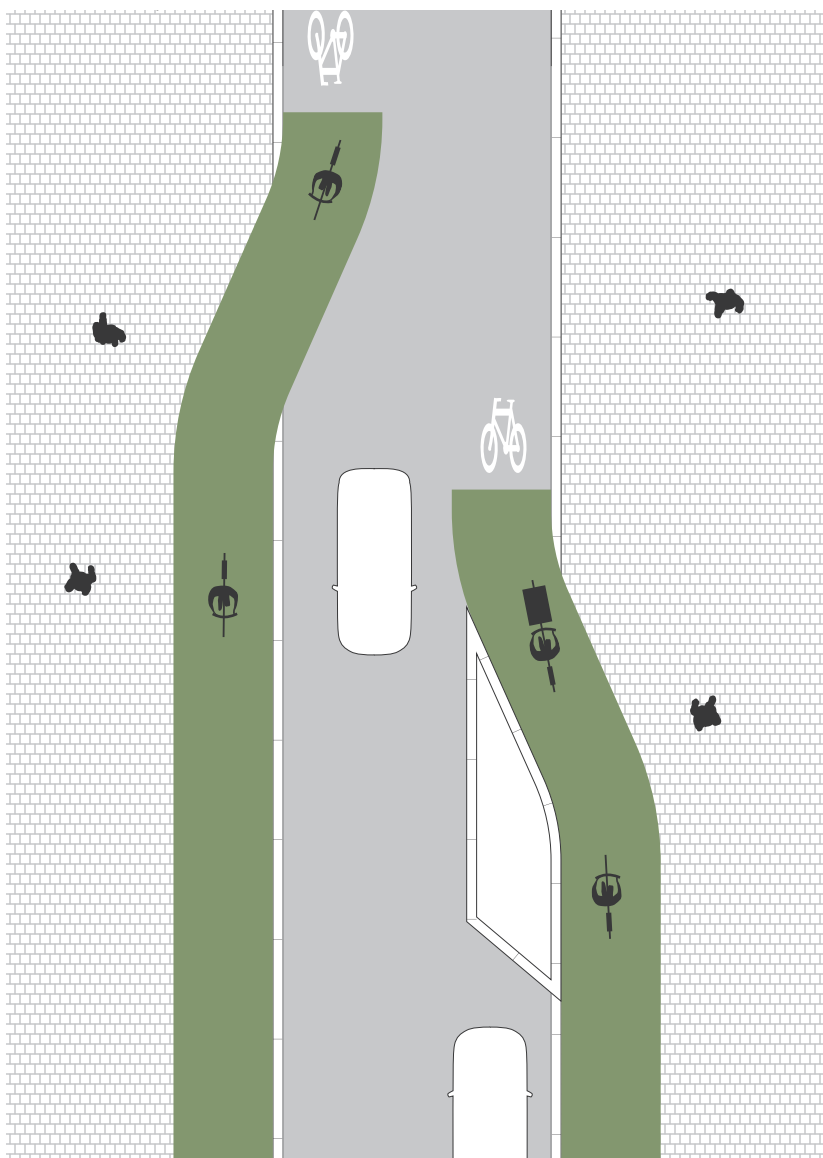
Fig. 1: Overgang naar gemengd verkeer met wegversmalling
