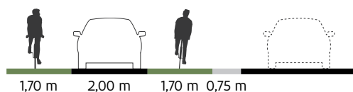
Voorbeeld 1: wegbreedte 5,40 m met een aanliggende parkeerstrook
