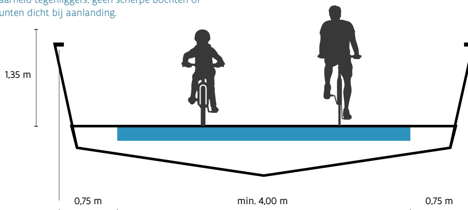
Fig. 1: Fietsbrug
