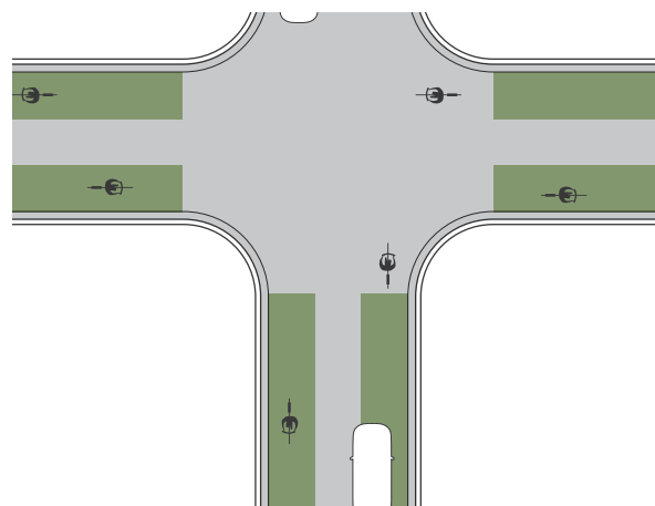
Fig. 3: Onderbroken fietssuggestiestrook bij voorrang van rechts
