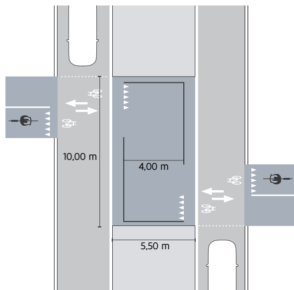
Fig. 4: Tweerichtingsfietsoversteekplaats in bajonetvorm uit de voorrang
