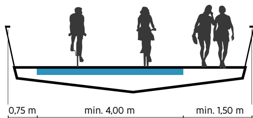
Fig. 2: Fietspad met voetpad aan één zijde
