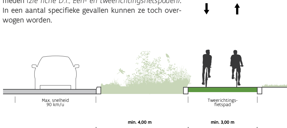
Fig. 3: Profiel tweerichtingsfietspad met een tussenstrook van 4,00 m bij een snelheidsregime van 90 km/u
