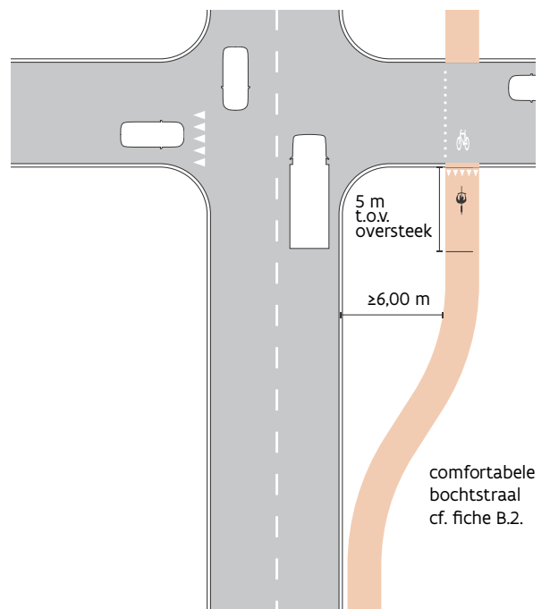
Fig. 6: Uitgebogen fietspad ( \geq 6,00 m) uit de voorrang
