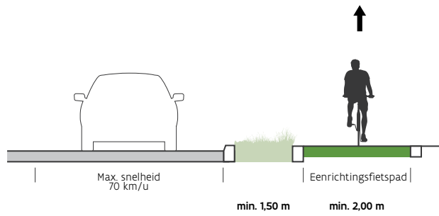
Fig. 1: Profiel vrijliggend eenrichtingsfietspad met een tussenstrook van 1,50 m bij een snelheidsregime van 70 km/u
