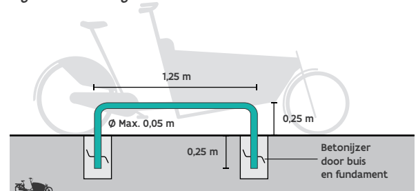
Fig. 4: Maatvoering buitenmaatse fietsen (ca. 10%)
