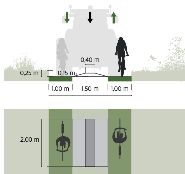
Fig. 1: Voorbehouden weg met tractorsluis
