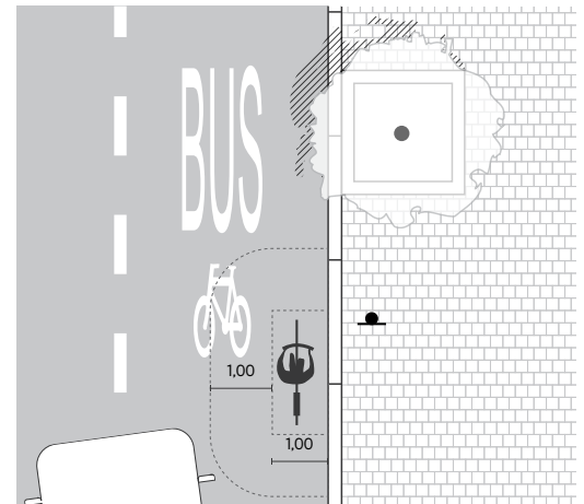
Fig. 4: busbaan met open profiel
