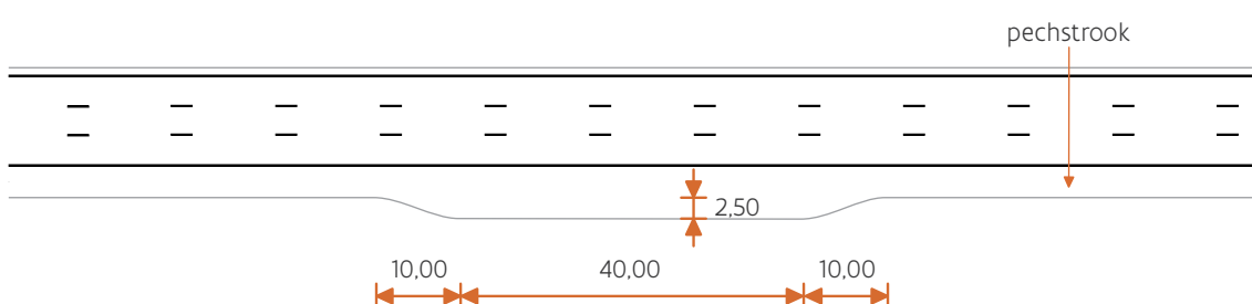
figuur 55: Pechhavens naast pechstrook op autosnelwegen
