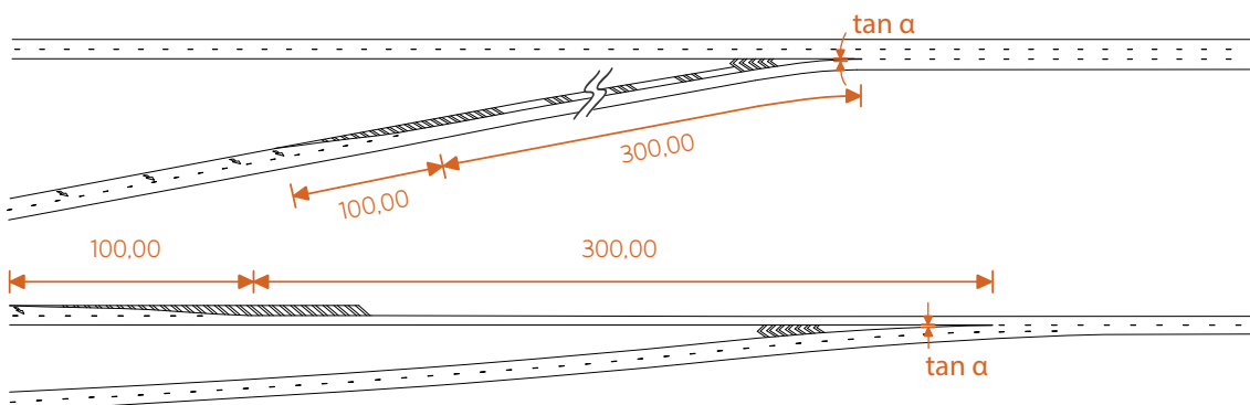
figuur 80: Samenvoeging met afnemend aantal rijstroken (De afmetingen in de afbeelding zijn gebaseerd op een ontwerpsnelheid van 120 km/h voor alle rijbanen)
