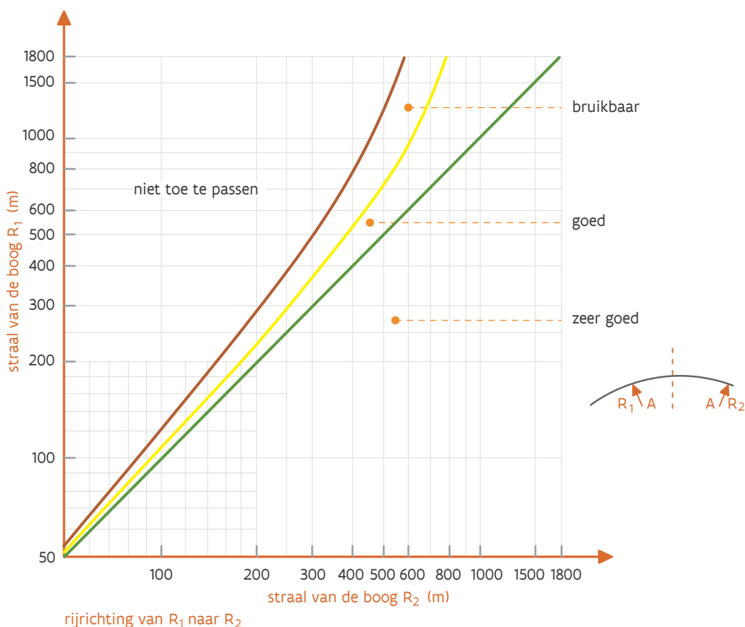
figuur 38: Toelaatbare stralen bij opeenvolgende gelijkgerichte horizontale bogen in niet-hoofdbanen (rijrichting van R_1 naar R_2 )
