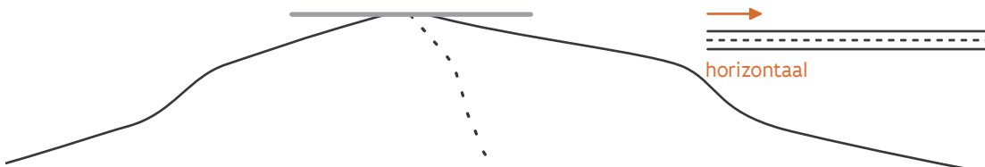
figuur 64: Verticale S-vorm met langshelling \geq 0,5\%
