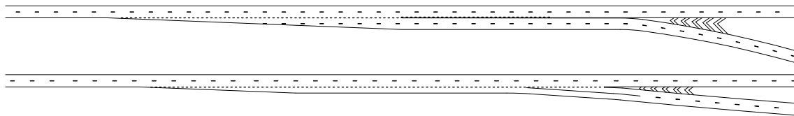
figuur 25: Principeschets tweestrookse uitvoeging (boven) en uitvoegende taper (onder)
