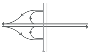
figuur 11: Halfklaverbladaansluiting
