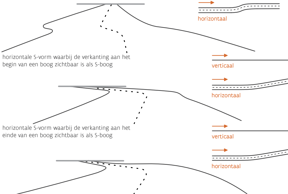
figuur 63: Horizontale S-vorm
