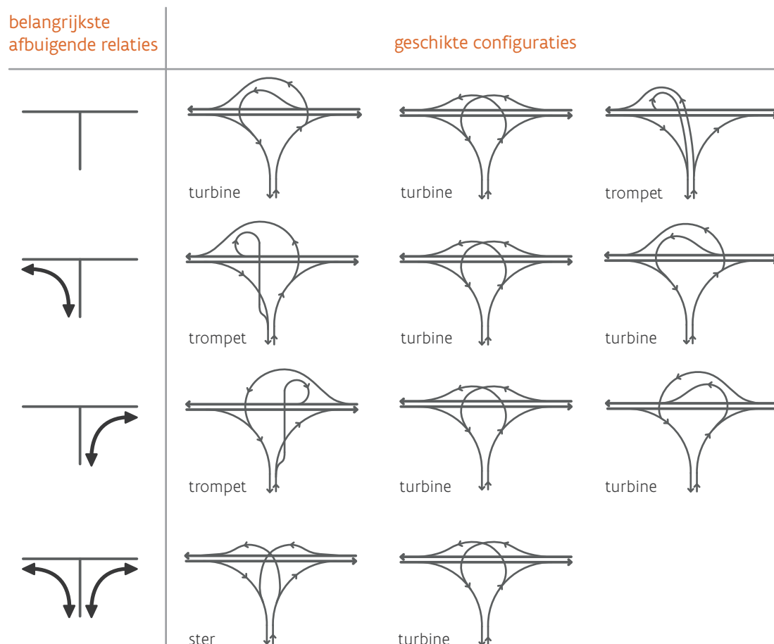
figuur 7: Standaard driearmige knooppuntconfiguraties
