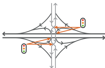
figuur 16: Aansluiting met een gevlochten Hollands complex
