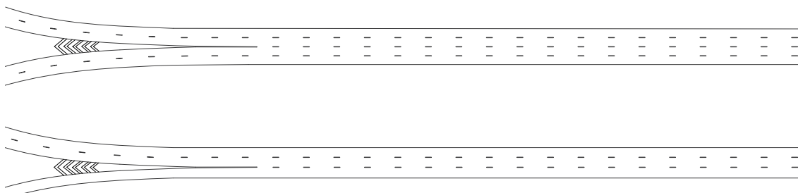
figuur 26: Principeschets standaard (zuivere) samenvoeging
