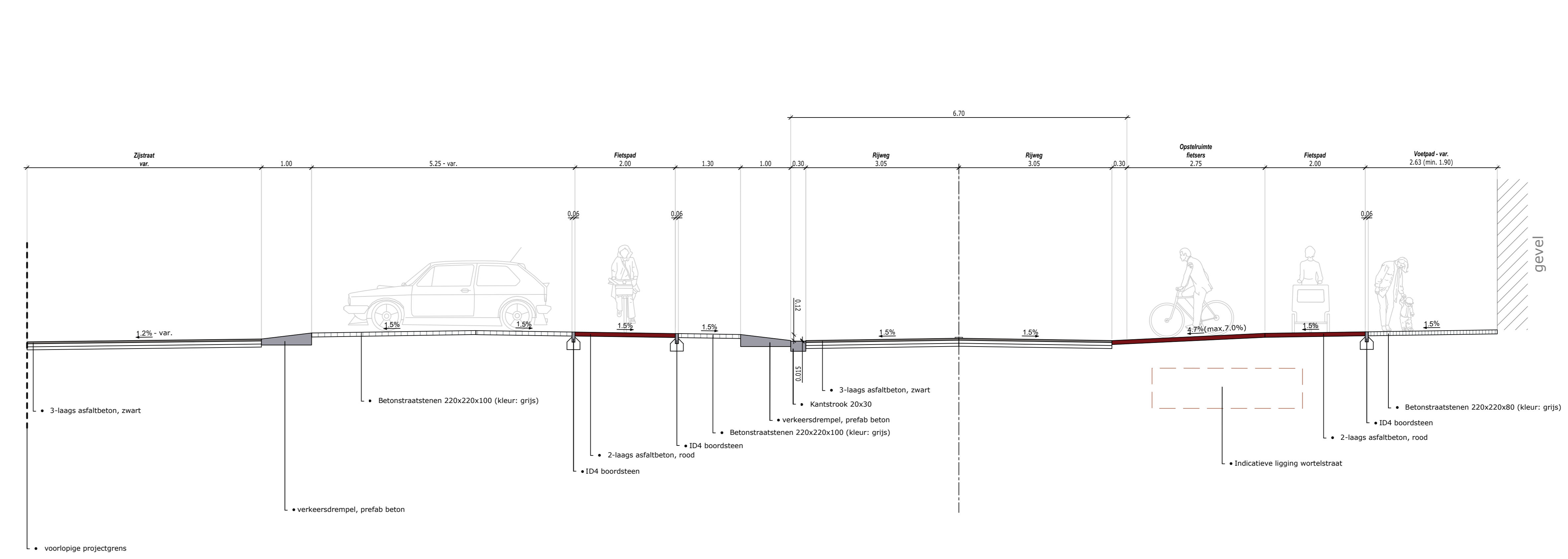
Typedwarsprofiel - Algemeen principe - zijstraat / fietsoversteek
