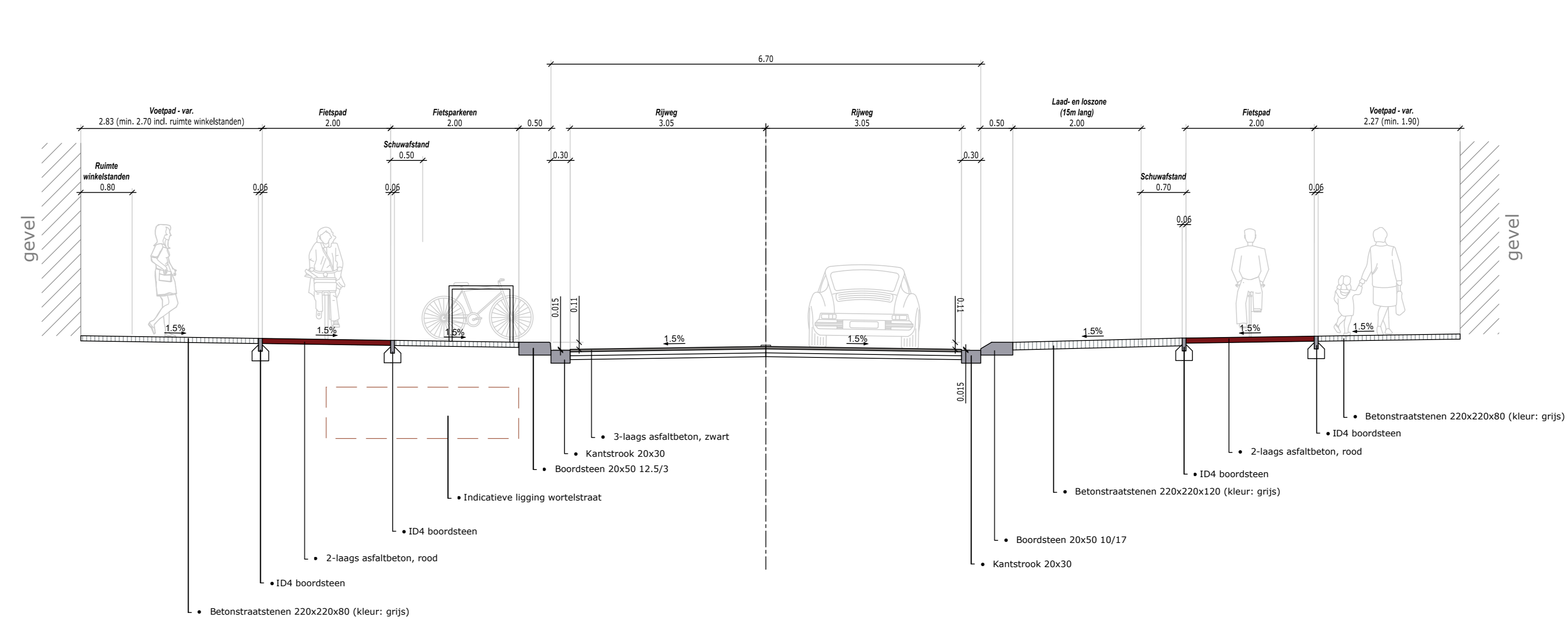
Typedwarsprofiel - Algemeen principe - fietsparkeren / laden en lossen (15m lang)
