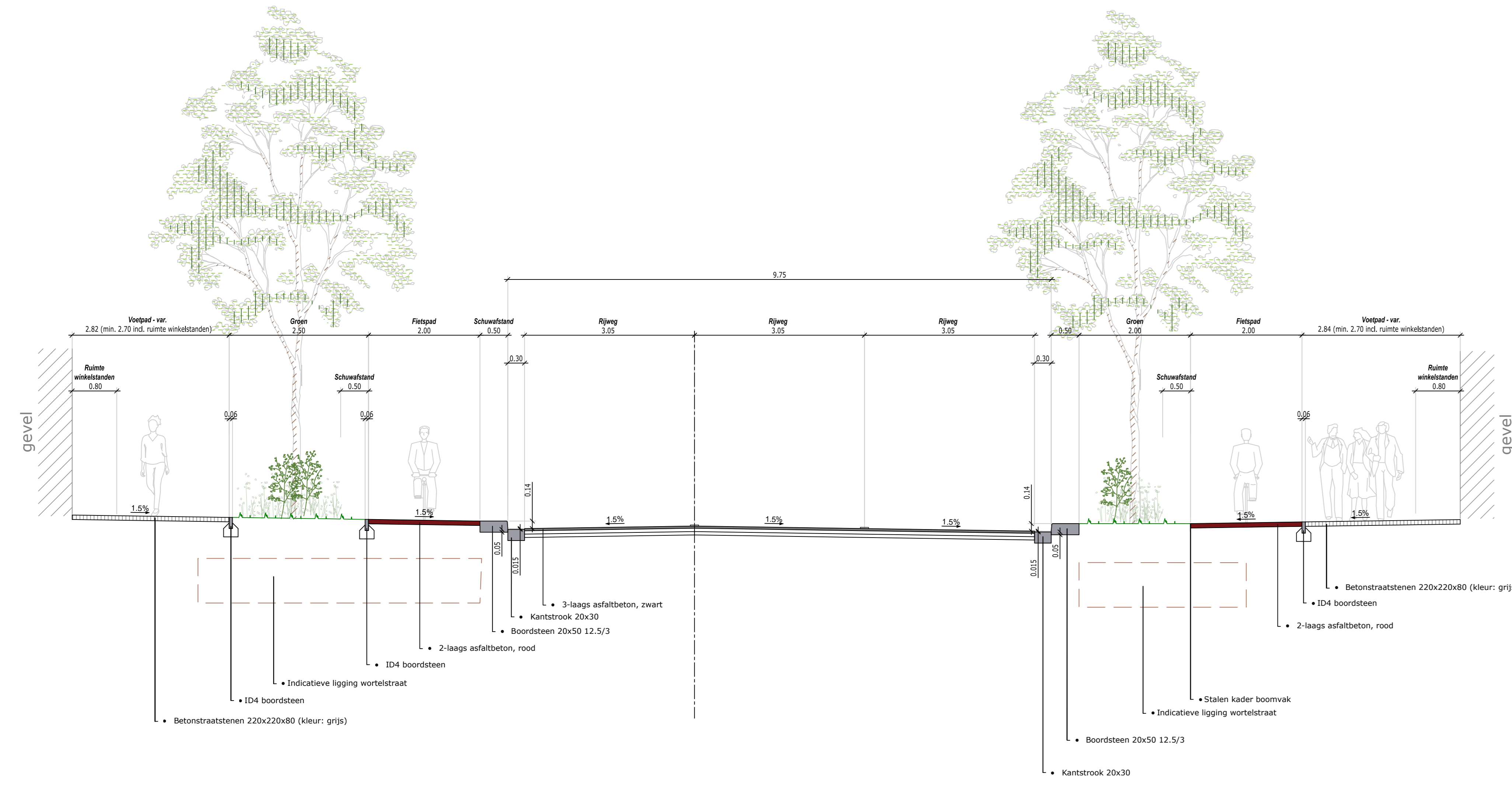
Typedwarsprofiel - SAS Provinciestraat - Kerkstraat - Algemeen principe - open plantvak/boomvak
