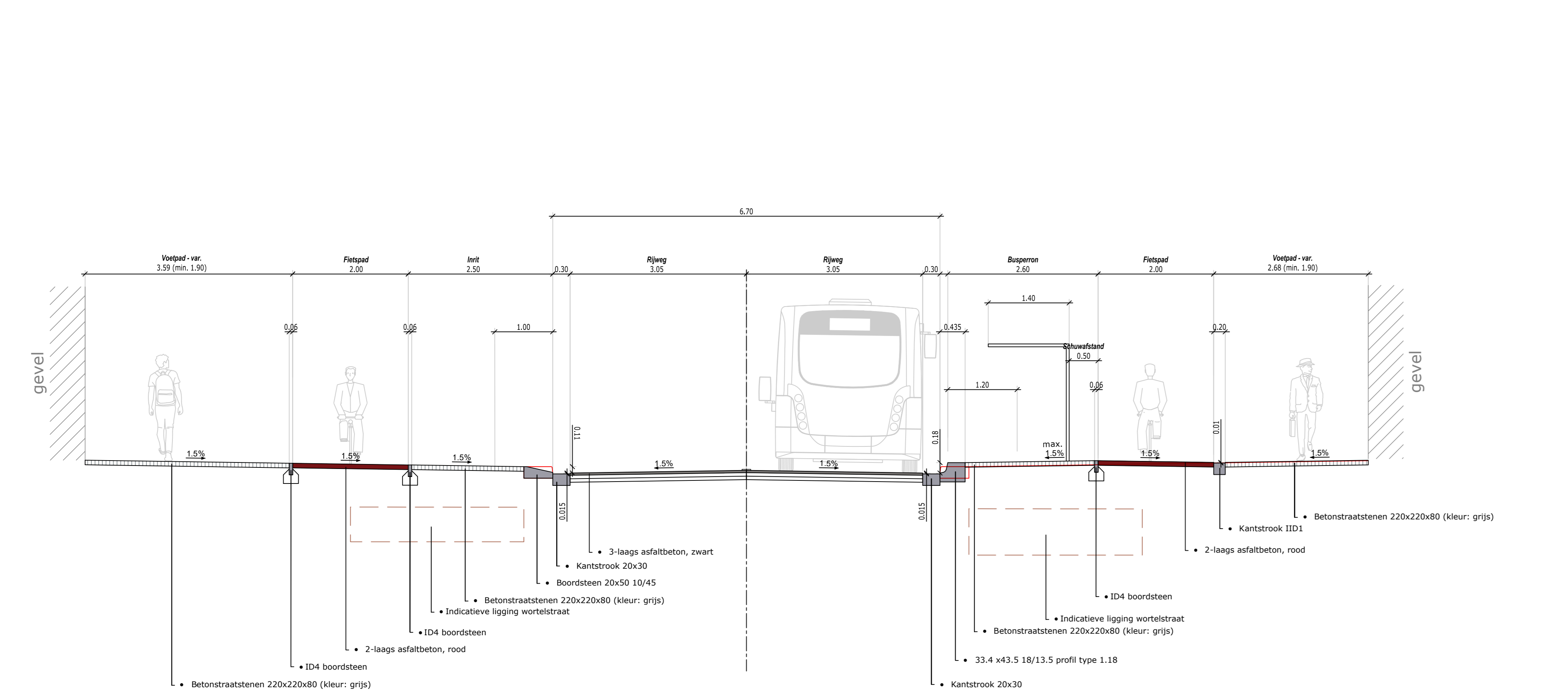
Typedwarsprofiel - Algemeen principe - inrichting achterliggende garages / bushalte
