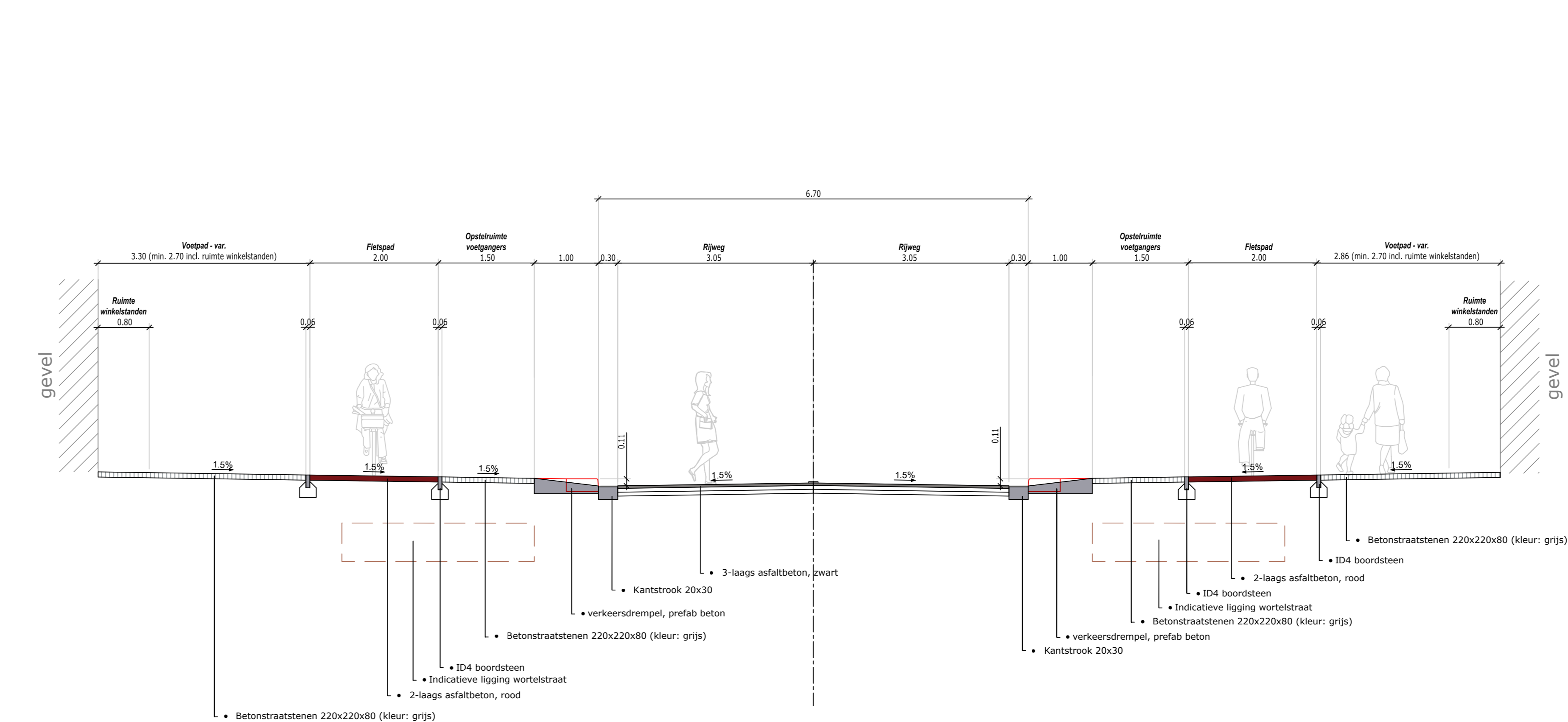
Typedwarsprofiel - Algemeen principe - voetgangersoversteek
