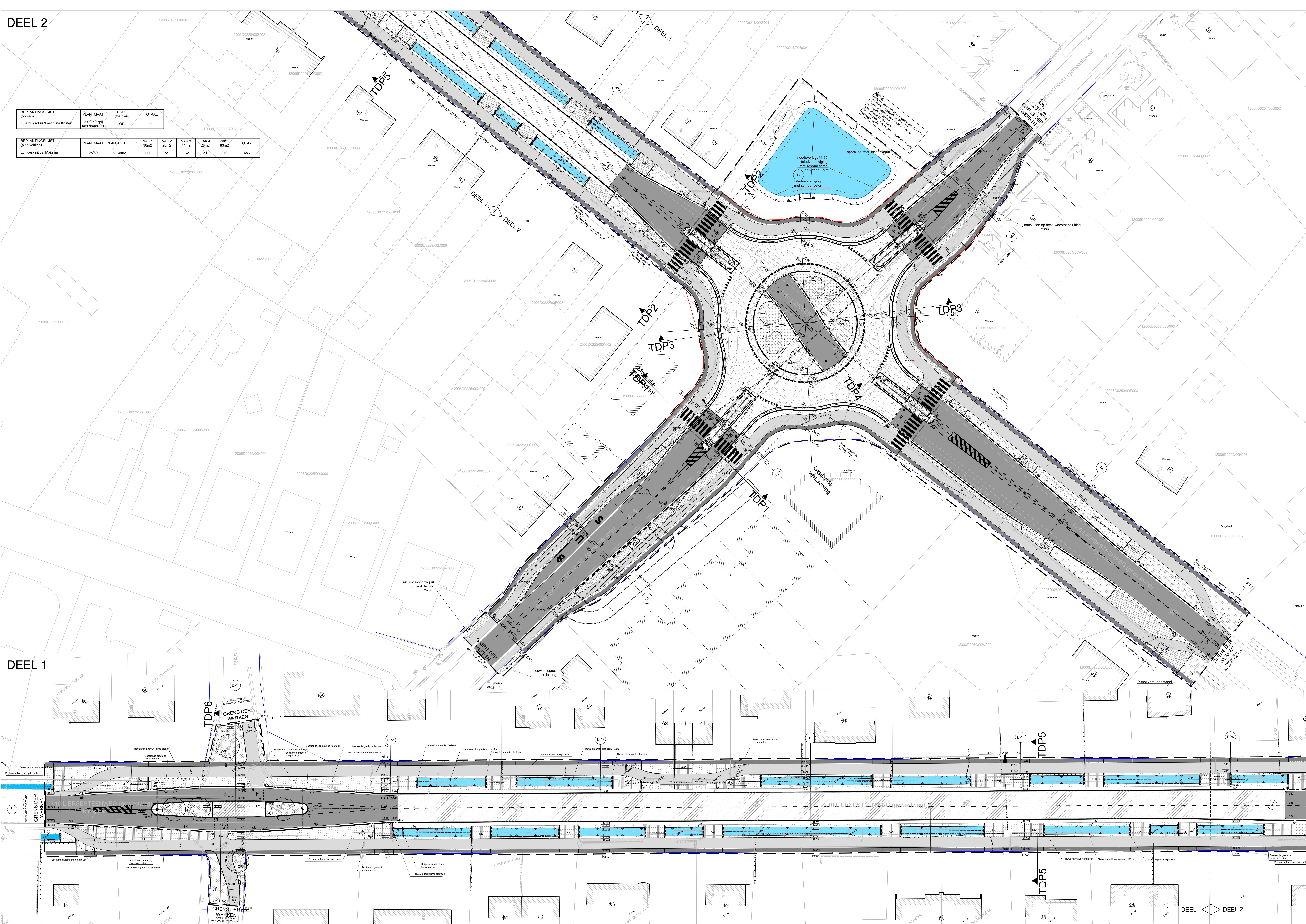
OVERZICHTSPLAN schaal : 1 / 2500
