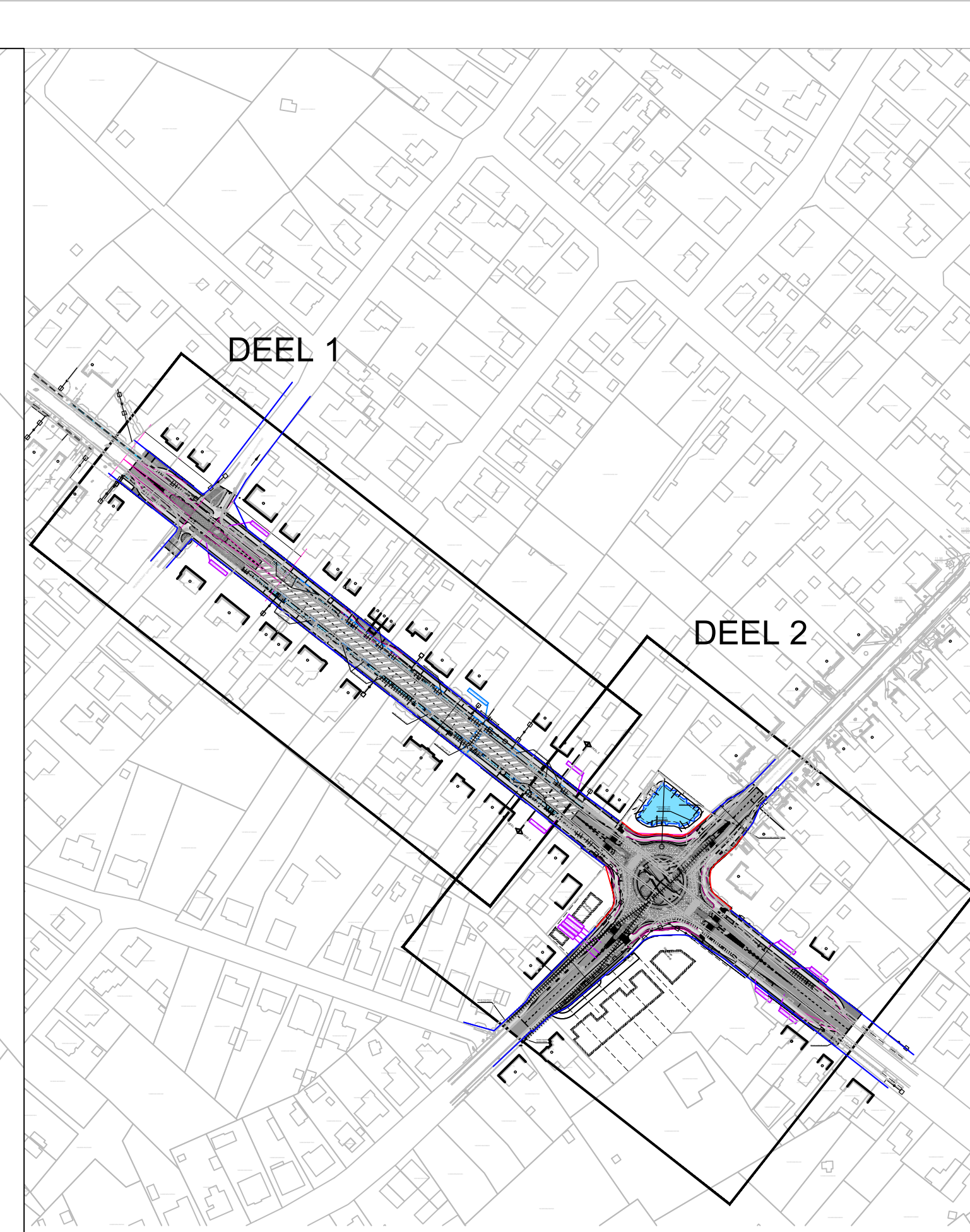
OVERZICHTSPLAN schaal : 1 / 2500
