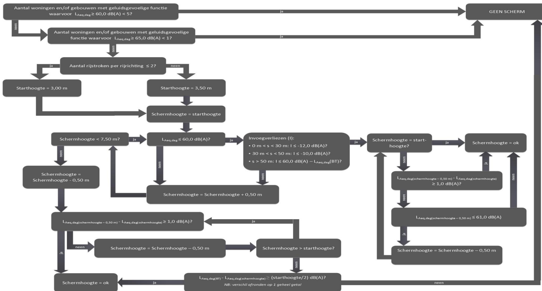
Figuur A: Stroomschema ter bepaling van de meest optimale hoogte van geluidswerende constructies
