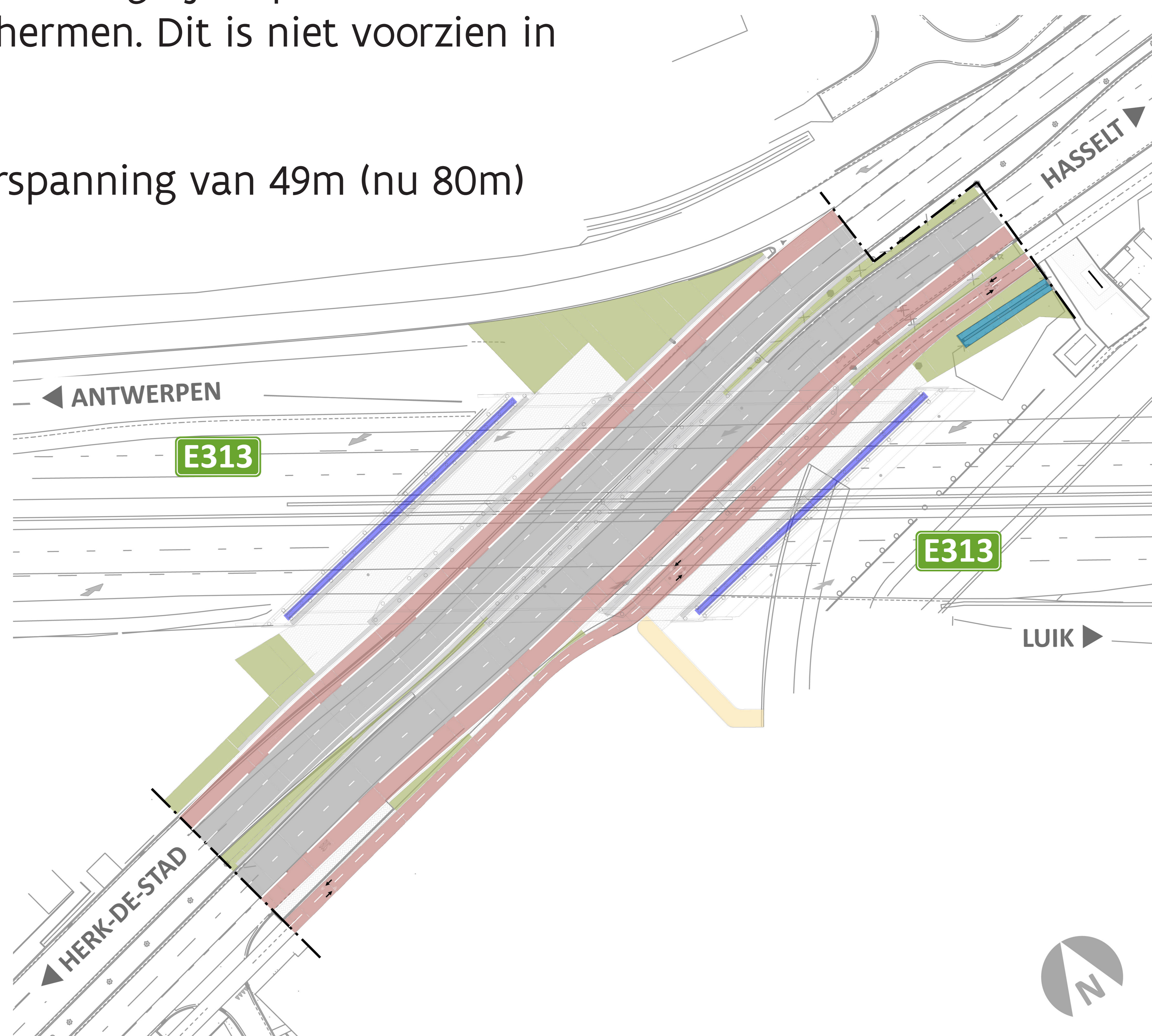
Grondplan Kuringersteenweg.
