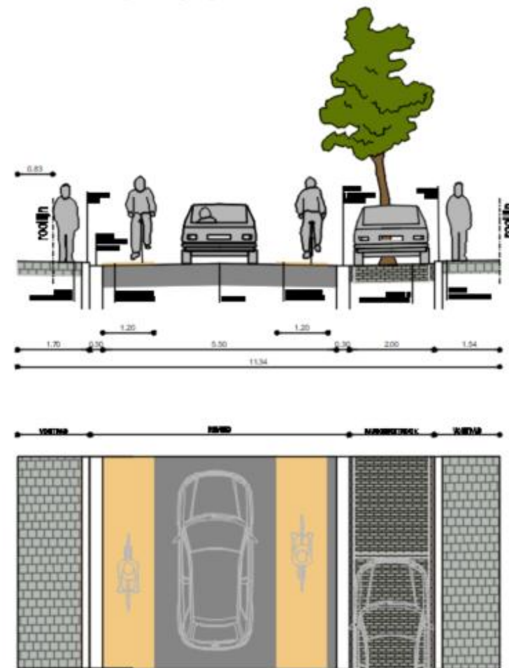
N347 Poperinge profil CC - Variant 3b
