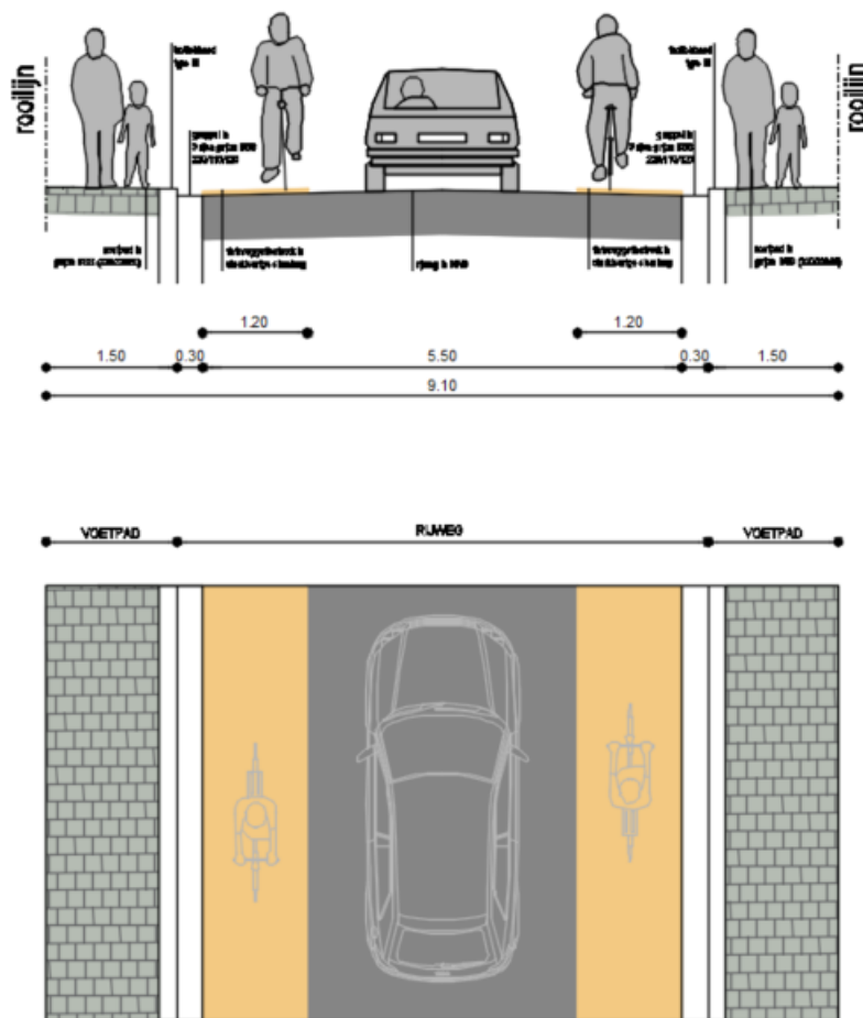
N347 Poperinge profil CC - Variant 3a
