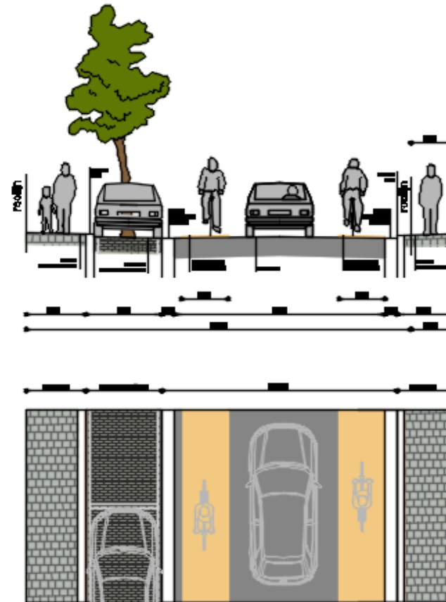
N347 Poperinge profiel GG
