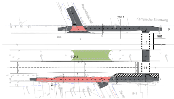
Ontwerpschets fietsoversteekplaats Kempische Steenweg
