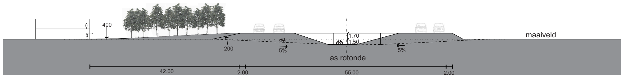
Lengteprofiel rotonde Potaardestraat
