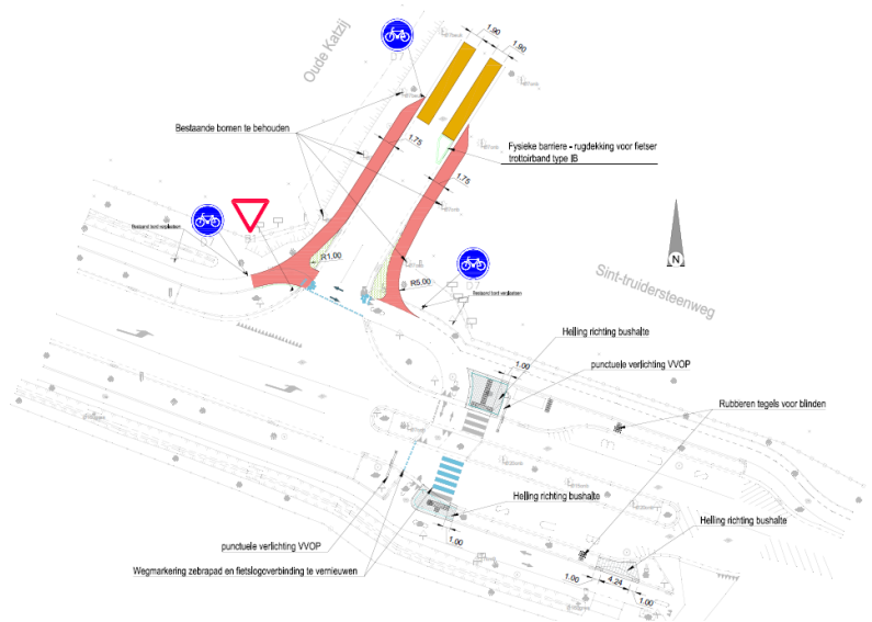
Schetstekening van de Sint-Truidersteenweg x Oude Katzij
