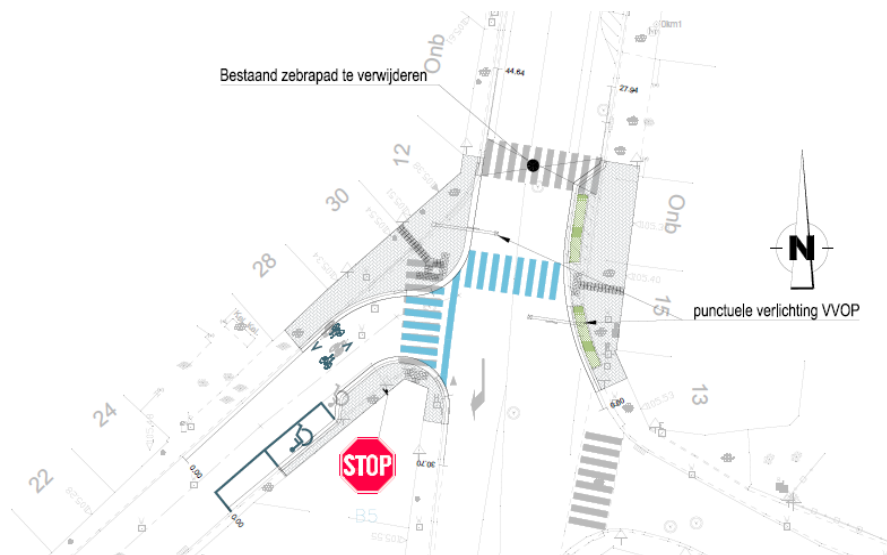
Schetstekening van het kruispunt Bilzersteenweg x Keversstraat
