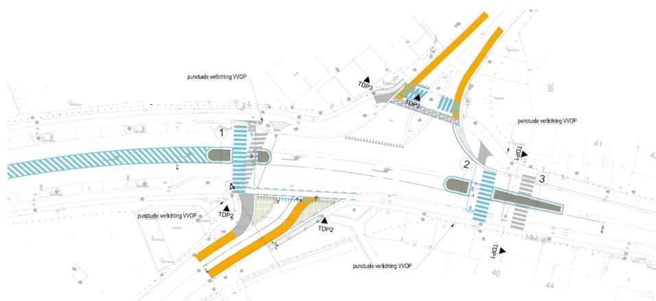
Schetstekening Heppensesteenweg x Pompstraat/Beukenlaan
